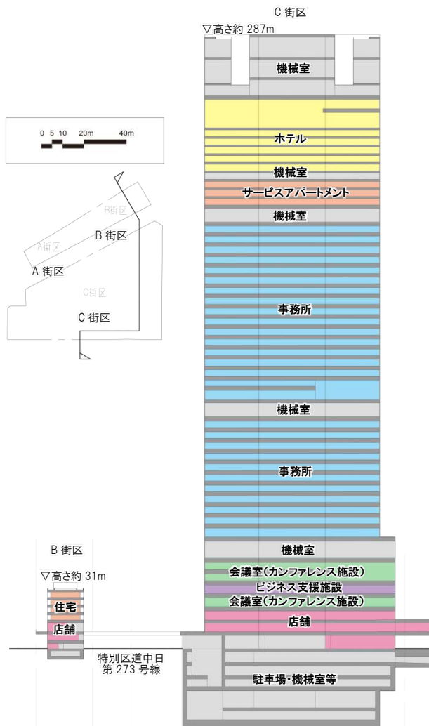
□断面図
