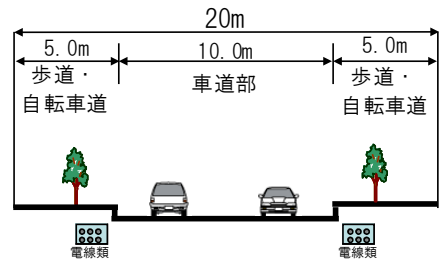
計 画 断 面 図（立体交差部）
