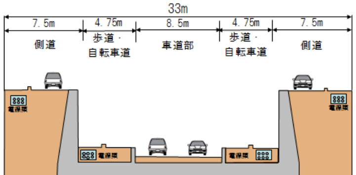
計 画 断 面 図（立体交差部）
