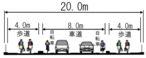
計画断面図
