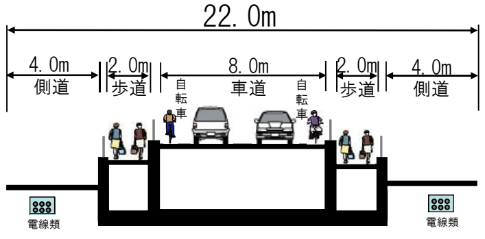
計画断面図
