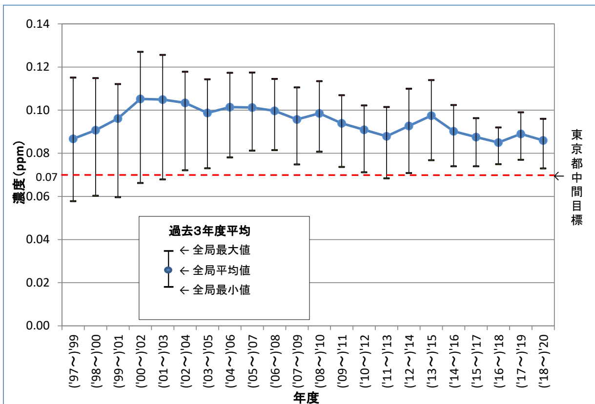
図5 年間4番目に高い日最高8時間値の3年平均の経年変化
