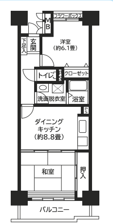
間取り図
