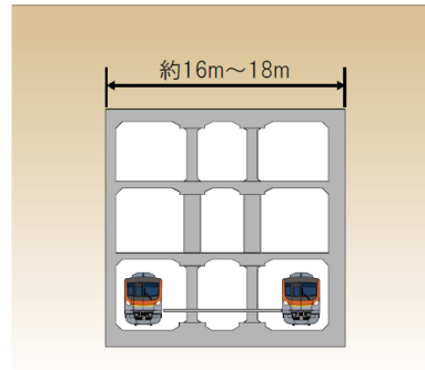
駅 間 部
