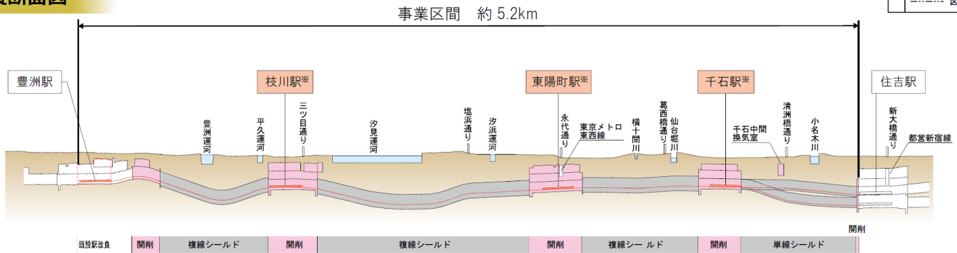
縦断面図
