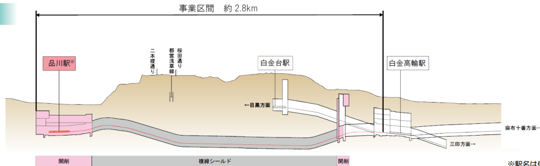
縦断面図
